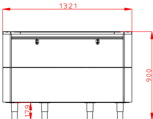
Alzado
